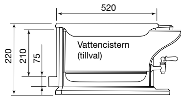
Vy från sidan
