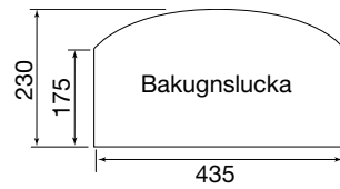
Vy bakifrån
