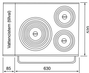
Vy uppfifrån bakanslutning
