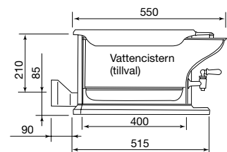
Vy från sidan
