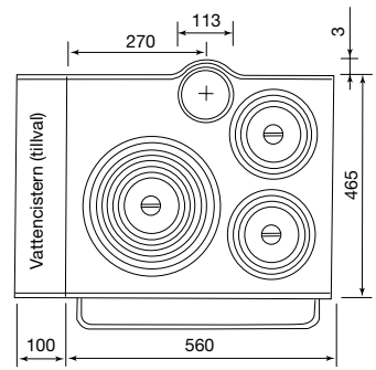
Vy uppfifrån toppanslutning
