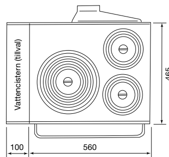
Vy uppfifrån bakanslutning
