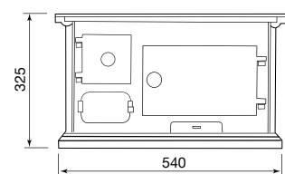
Vy framifrån
